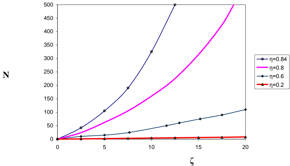
الشكل رقم 3-b يوضح العلاقة بين مظاهر مختلفة لكثافات البلازما المحورية عند \sigma=1.23 , \gamma=0.85 , ومختلف القيم لسمك القضيب المعدني \zeta
