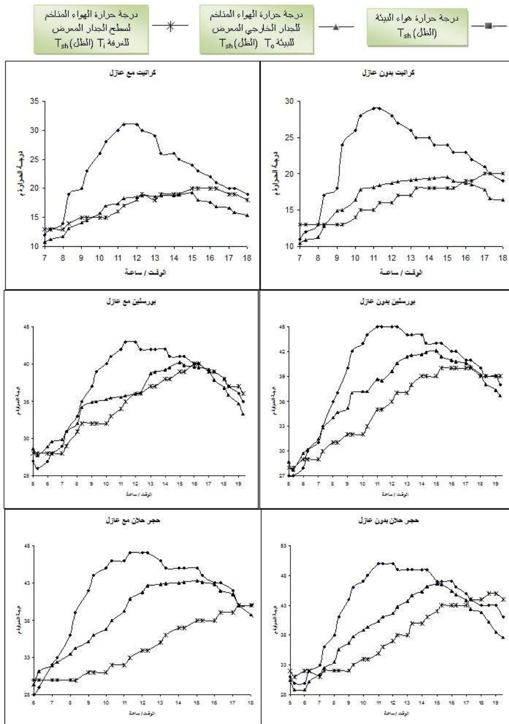
شكل (5) الأداء الحراري للجدار المغلف من الداخل بمواد الكرايتيت والبورسلين وحجر الحلان بوجود
