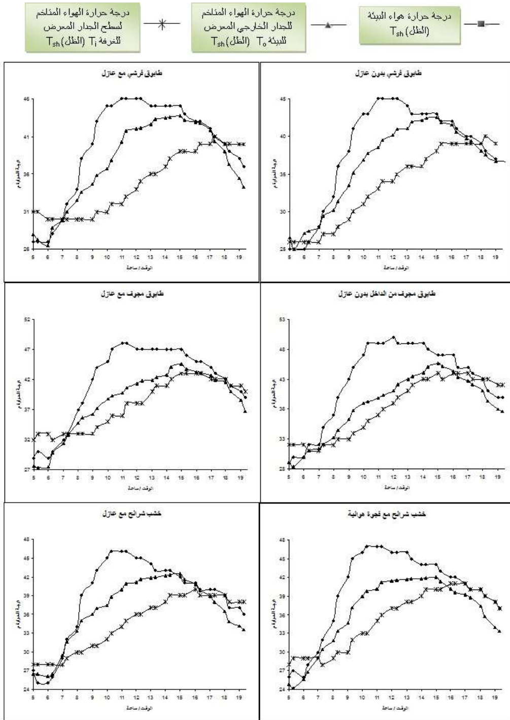
شكل (6) الأداء الحراري للجدار المغلف من الداخل بمواد الطابوق القرشي والطابوق المجوف وخشب شرائح
