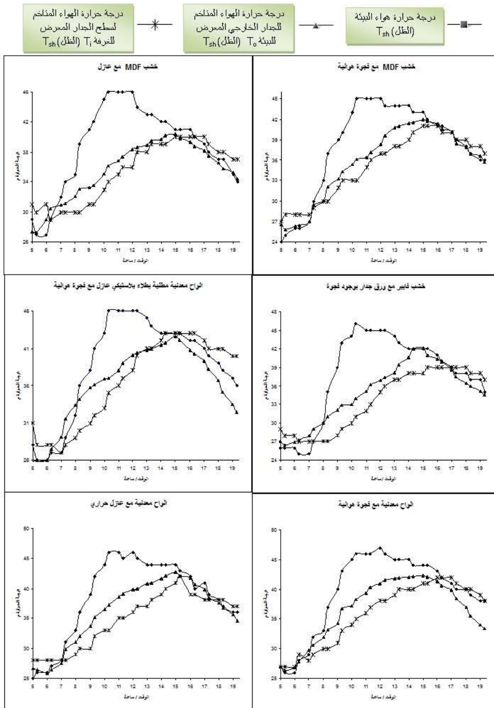
شكل (7) الأداء الحراري للجدار المغلف من الداخل بمواد خشب MDF وخشب فايبر وأواح معنبة مطلية بطلاء بلاستيكي
