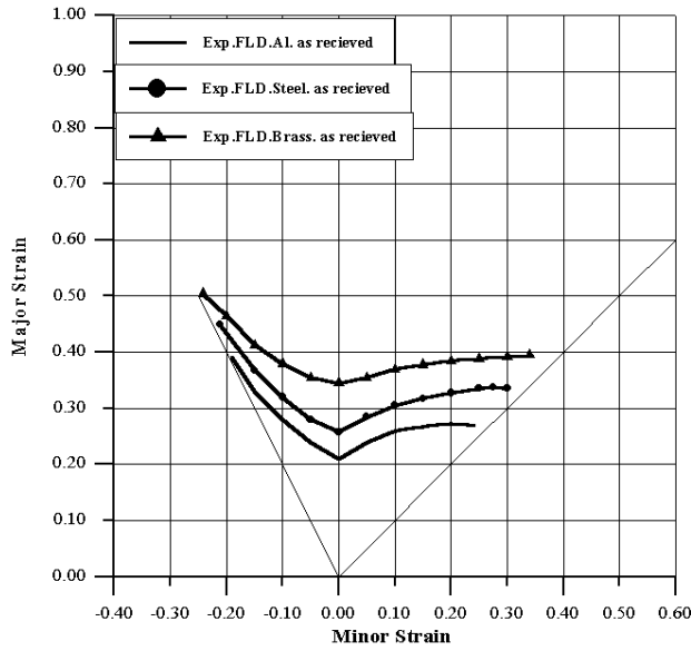
شكل (8) منحنى حد التشكيل للألمنيوم والصلب والبراص
