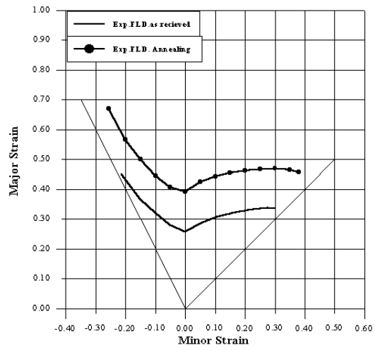
شكل (14) يبين تأثير التلدين على منحنى الصلب
