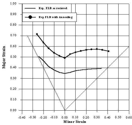
شكل (15) يبين تأثير التلدين على منحنى البراص
