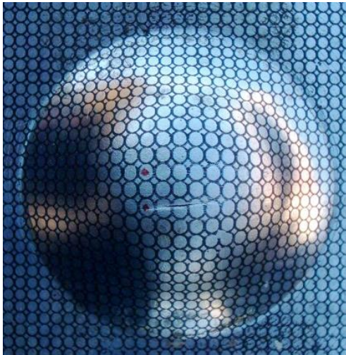
شكل(6) النموذج (8) من الألمنيوم بعد التشكيل
