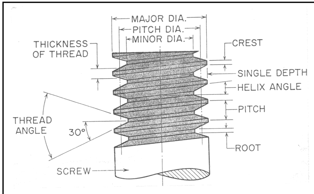
شكل رقم (1) يبين رسماً توضيحياً لشكل وأبعاد المحيط الأساسي لأسنان المسامير الملولبة (النظام المتري) [7].
