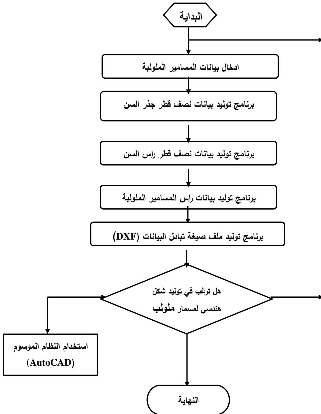
شكل رقم (3) يبين رسماً تخطيطياً للمخطط الكلي للبرامج المكونة للنظام المقترح
