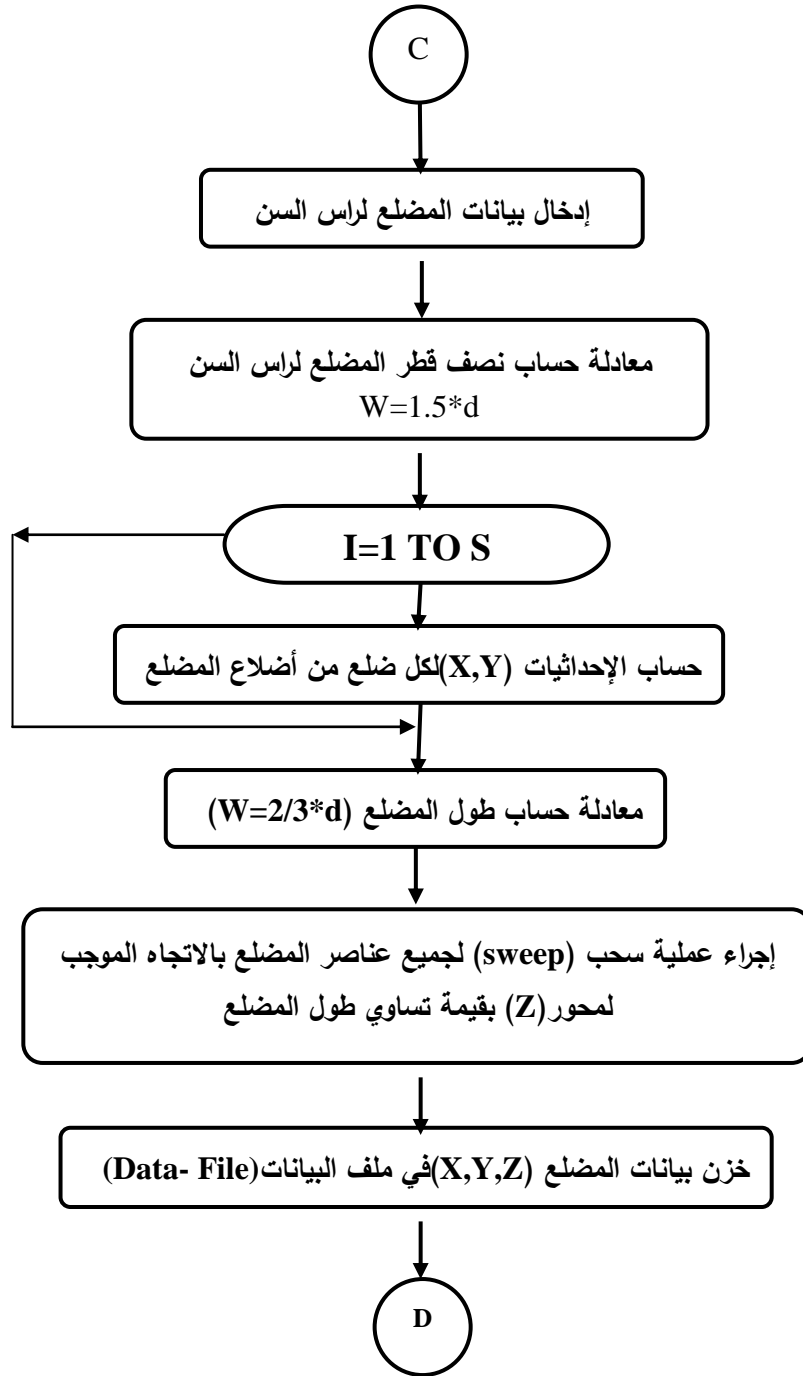
شكل رقم (6) يبين المخطط الانسيابي لخوارزمية حساب التصميم الهندسي لرأس المسامير الملولبة.
