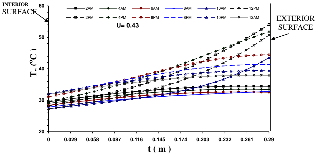
شكل ( 5 ) توزيع درجات الحرارة في جدار ترومب مغطى سطحه الخارجي بطبقتين
