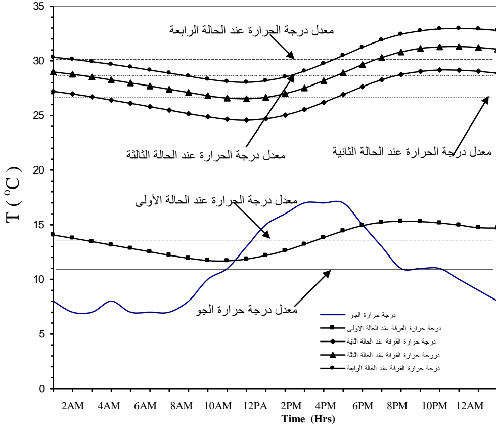
شكل (7) تغير درجات الحرارة لكل من درجة حرارة الجو ودرجة حرارة الغرفة المكيفة بجدار ترอมب للحالات الأربعة مع الزمن تحت الظروف المناخية لمدينة بغداد ليوم
