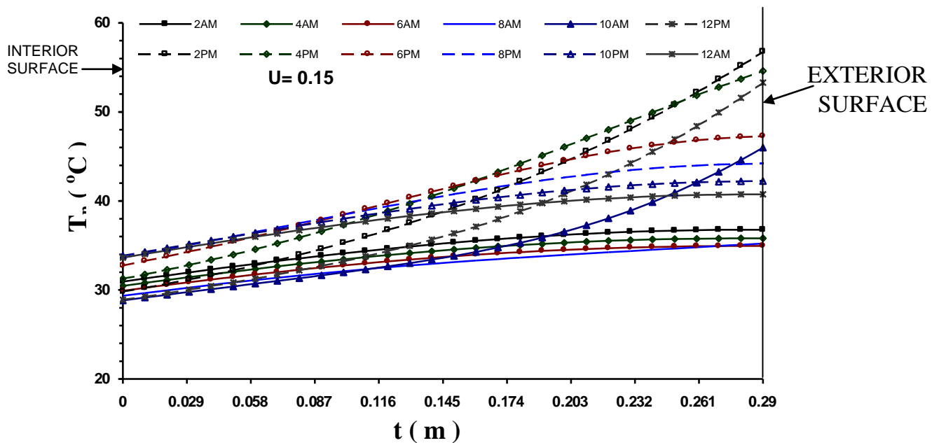
شكل ( 6 ) توزيع درجات الحرارة في جدار ترومب تغطي سطحه الخارجي بثلاث
