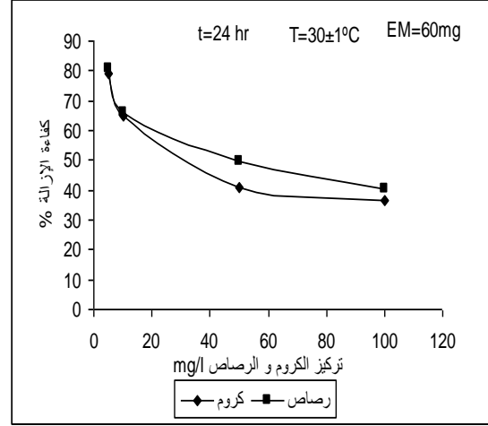
شكل (15) إنتقائية الأحياء المجرية الفعالة عند عند نسبة إضافة 60 ملغم ولمختلف تراكيز الكروم والرصاص
