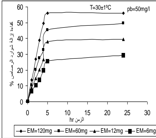
شكل (10) تغاير كفاءة إزالة الرصاص مع زمن التماس عند مختلف تراكيز الكتلة الحية المطبقة وتركيز أولي مقداره (50 ملغم/لتر)
