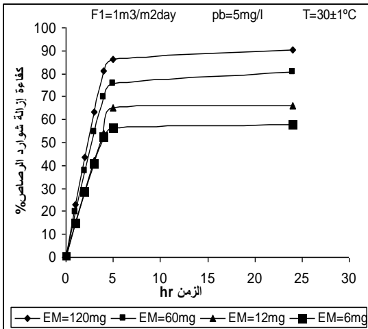
شكل (6) تغير كفاءة إزالة الرصاص مع زمن التماس عند مختلف تراكيز الكتلة الحية المطبقة وتركيز أولي مقداره (5 ملغم/لتر)
