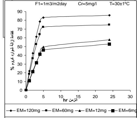
شكل (5) تغير كفاءة إزالة الكروم مع زمن التماس عند مختلف تراكيز الكتلة الحية المطبقة وتركيز أولي مقداره (5 ملغم/لتر)
