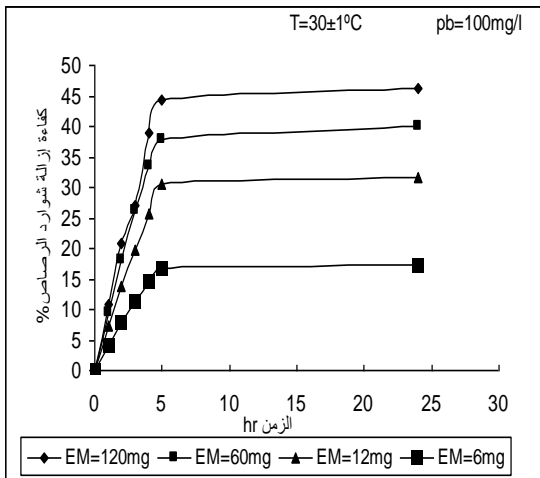
شكل (12) تغاير كفاءة إزالة الرصاص مع زمن التماس عند مختلف تراكيز الكتلة الحية المطبقة
