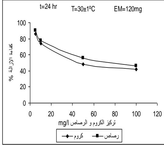
شكل (16) إنتقائية الأحياء المجرية الفعالة عند عند نسبة إضافة 120 ملغم ولمختلف تراكيز الكروم والرصاص
