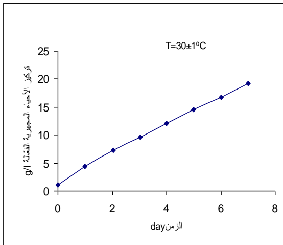
شكل رقم (1) يوضح تركيز الأحياء المجهرية مع زمن الأقلمة
