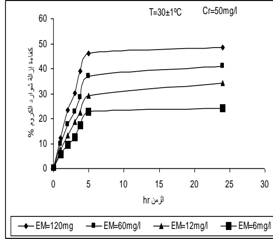
شكل (9) تغاير كفاءة إزالة الكروم مع زمن التماس عند مختلف تراكيز الكتلة الحية المطبقة وتركيز أولي مقداره (50 ملغم/لتر)
