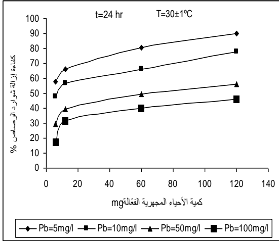
شكل (4) كفاءة إزالة الرصاص عند مختلف التراكيز الابتدائية ومختلف تراكيز الكتلة الحية المطبقة
