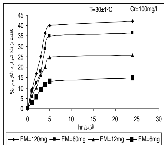
شكل (11) تغاير كفاءة إزالة الكروم مع زمن التماس عند مختلف تراكيز الكتلة الحية المطبقة
