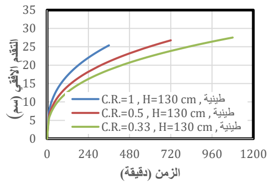
الشكل (6): العلاقة بين تقدم الابتلال الأفقي مع الزمن لنسب الدورة 1 و 0.5 و 0.33
