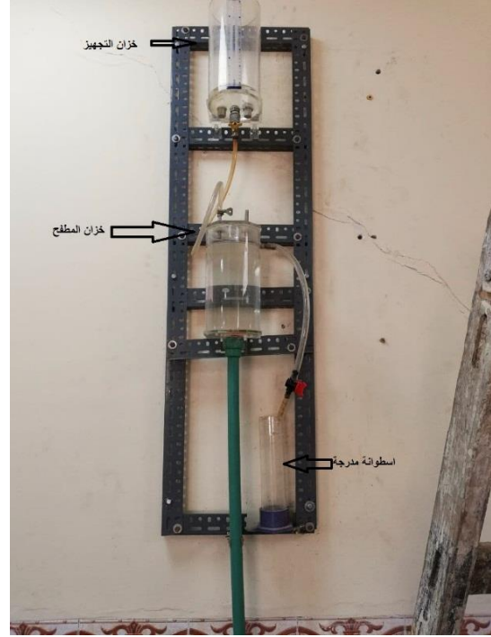
الشكل (2): منظومة تجهيز المنقط بالماء
