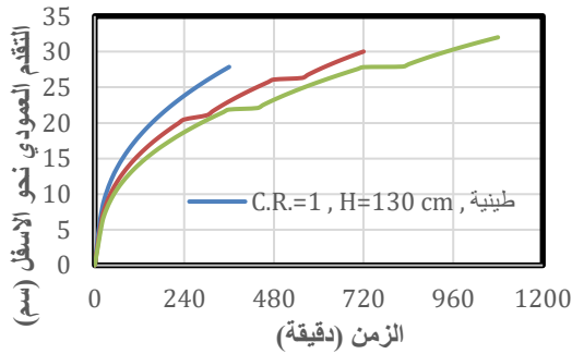
الشكل (8): العلاقة بين تقدم الابتلال العمودي نحو الاسفل مع الزمن لنسب الدورة 1 و 0.5 و 0.33
