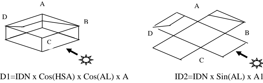
الشكل (7) طريقة حساب كفاءة التعرض الشمسي للفناءات
