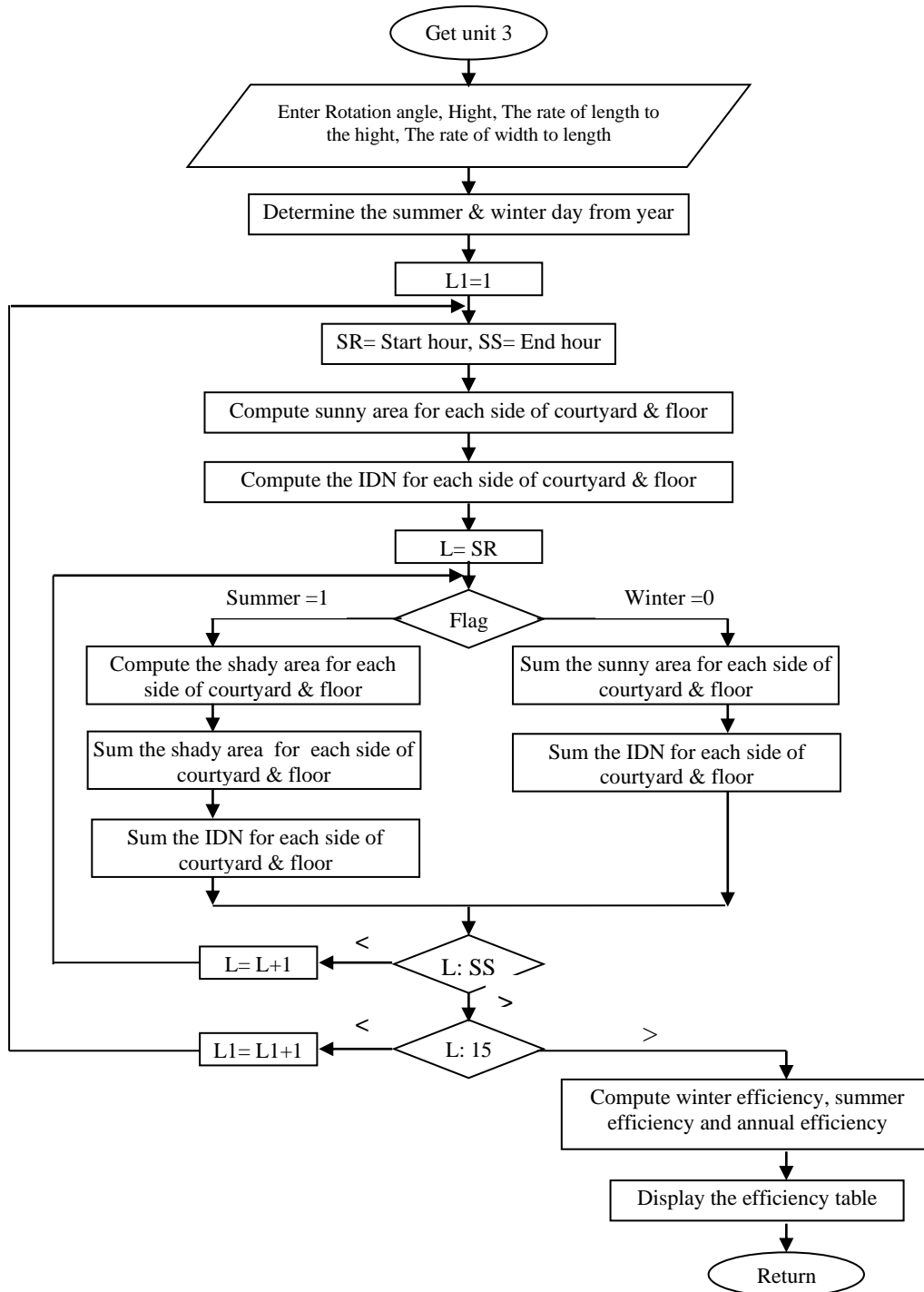
الشكل (11) المخطط الانسيابي لوحدة حساب كفاءة الفناء
