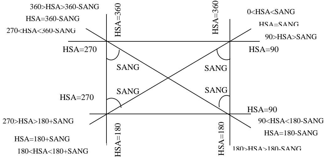
الشكل (10) اتجاه نفوذ الأشعة الشمسية حسب قيمة زاوية الظل الأفقية (HSA)
