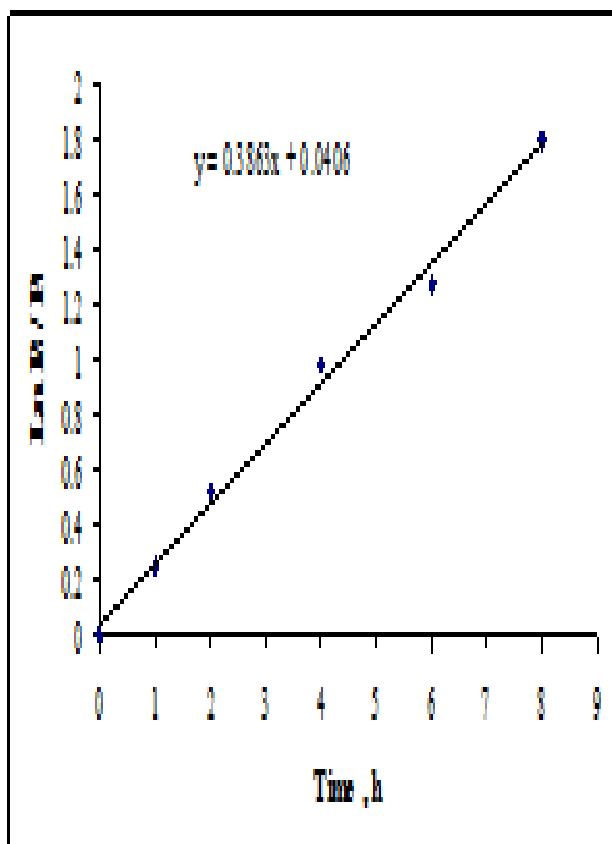
شكل (4) سرعة تحلل مبيد Actellic بدرجة حرارة 313 مطلقه
