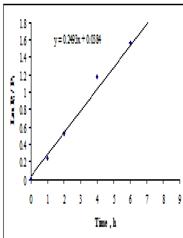
شكل (2) سرعة تحلل مبيد Actellic بدرجة حرارة 283 مطلقه
