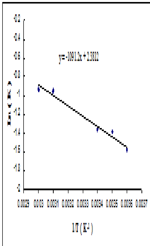
شكل (6) يبين تأثير درجة الحرارة في سرعة تحلل مبيد Actellic
