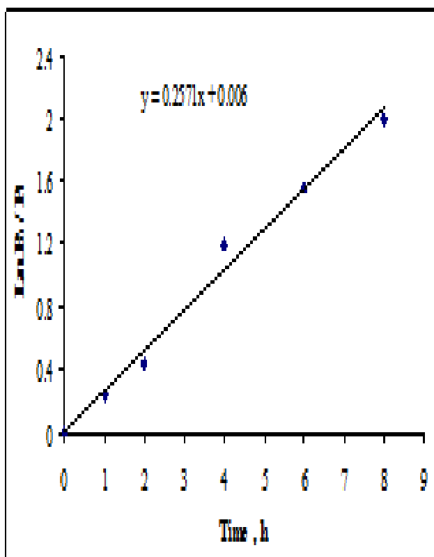
شكل (3) سرعة تحلل مبيد Actellic بدرجة حرارة 293 مطلقه
