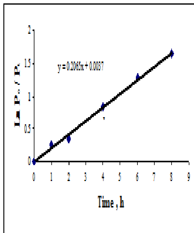
شكل (1) سرعة تحلل مبيد Actellic بدرجة حرارة 278 مطلقه
