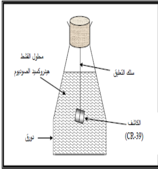
الشكل (2) طريقة تعليق الكاشف (CR-39) في محلول القشط -المعاينة المجهرية
