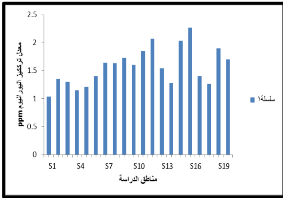
شكل (3) معدل تركيز اليورانيوم في ترب مناطق الدراسة لمدينة الفلوجة
