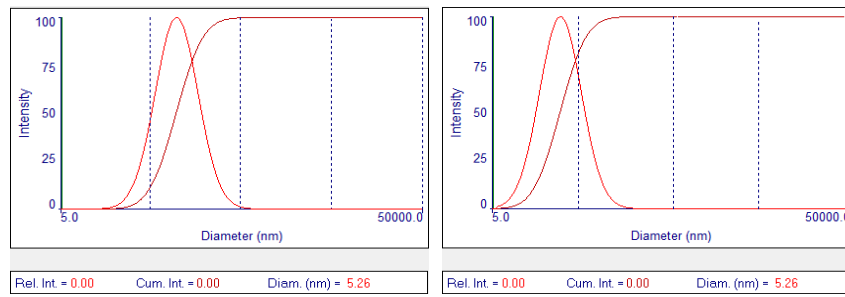
a. b. Figure (2) P.S Spectra of a: TiO 2 , b:CuO
